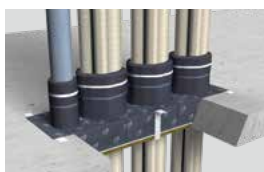
RC・ALC床（鋼製スリーブなし） PS060FL-1200
