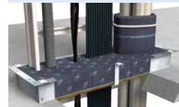
RC・ALC床 (鋼製スリーブあり) PS060FL-1200
